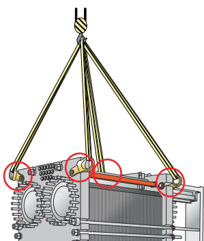
Figur 7: Løfteanordning til T50. Der skal bruges fastgøringsudstyr.
