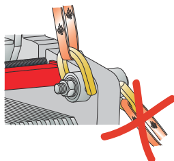
Figur 8: Løfteanordning til TS50. Benyt de fire indvendige løfteøjer til løft af pladevarmeveksleren. Brug IKKE transportøjerne! Der skal bruges fastgøringsudstyr.
