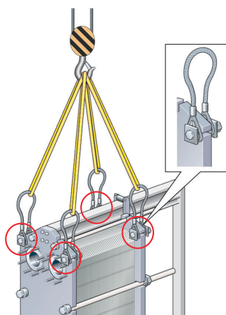
Figur 5: Løfteanordning til T35 og TS35. Der skal bruges fastgøringsudstyr.
